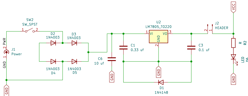
Power module
